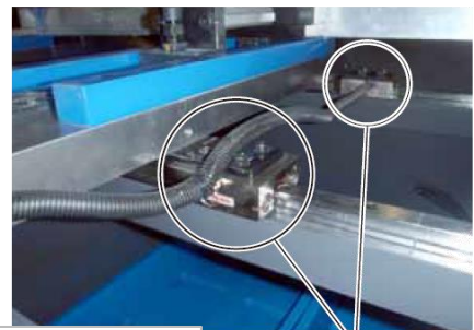
数控长尺加工机的虎钳
