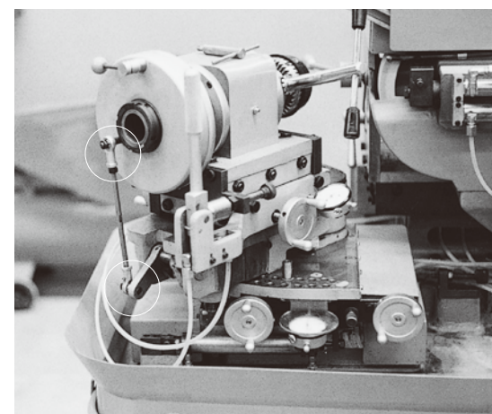
工具研磨機
