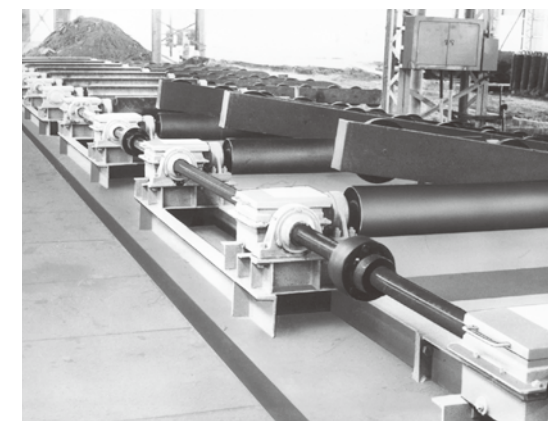
ローラガング
