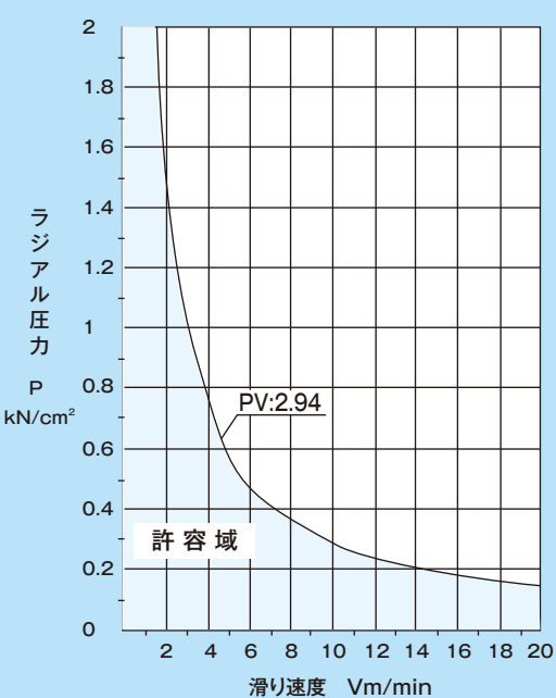
〈図5.3〉 ジョインボールの許容PV値
