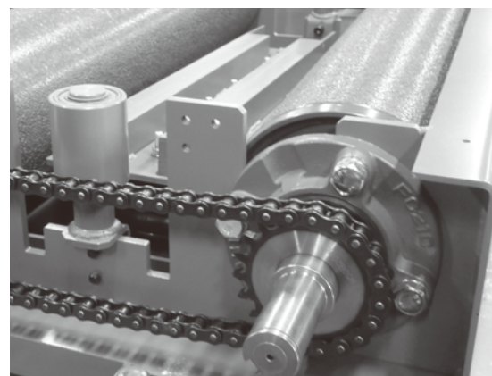
車検装置
