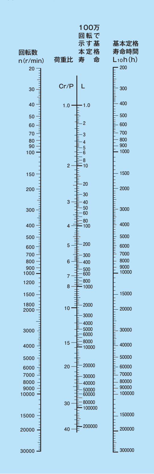
<図4.1> n-C_r/P_r-L_{10h} ノモグラフ
