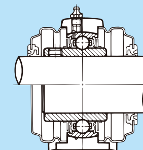
<図2>鋼板製カバー付きピロー形ユニットの断面図
