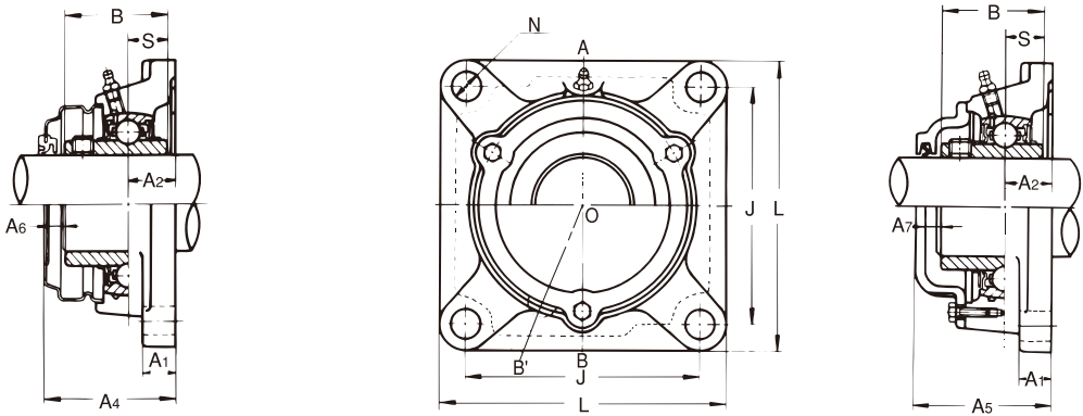
鋳鉄製カバー付き 断面AOB':CUCF200C(CE)形 断面AOB :CUCF300C(CE)形
