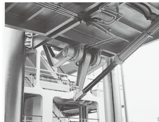
フェリー用タラップ
