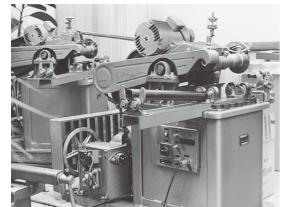
切 断 機
