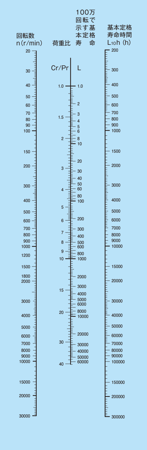
〈図4.5〉 n-Cr/Pr- L_{10h} ノモグラフ
