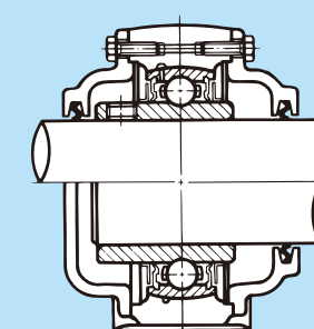
<図3>鋳鉄製カバー付きピロー形ユニットの断面図
